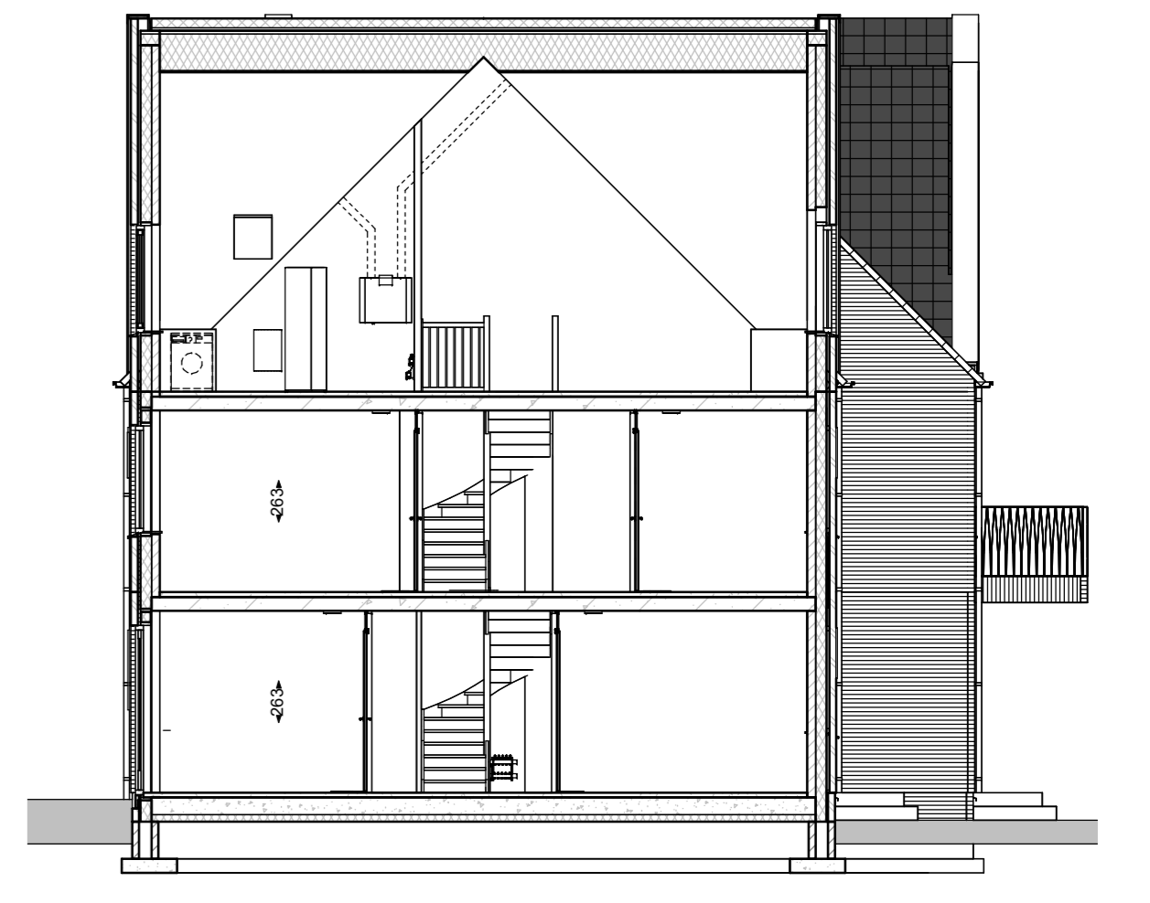
DOORSNEDE A schaal 1:100
