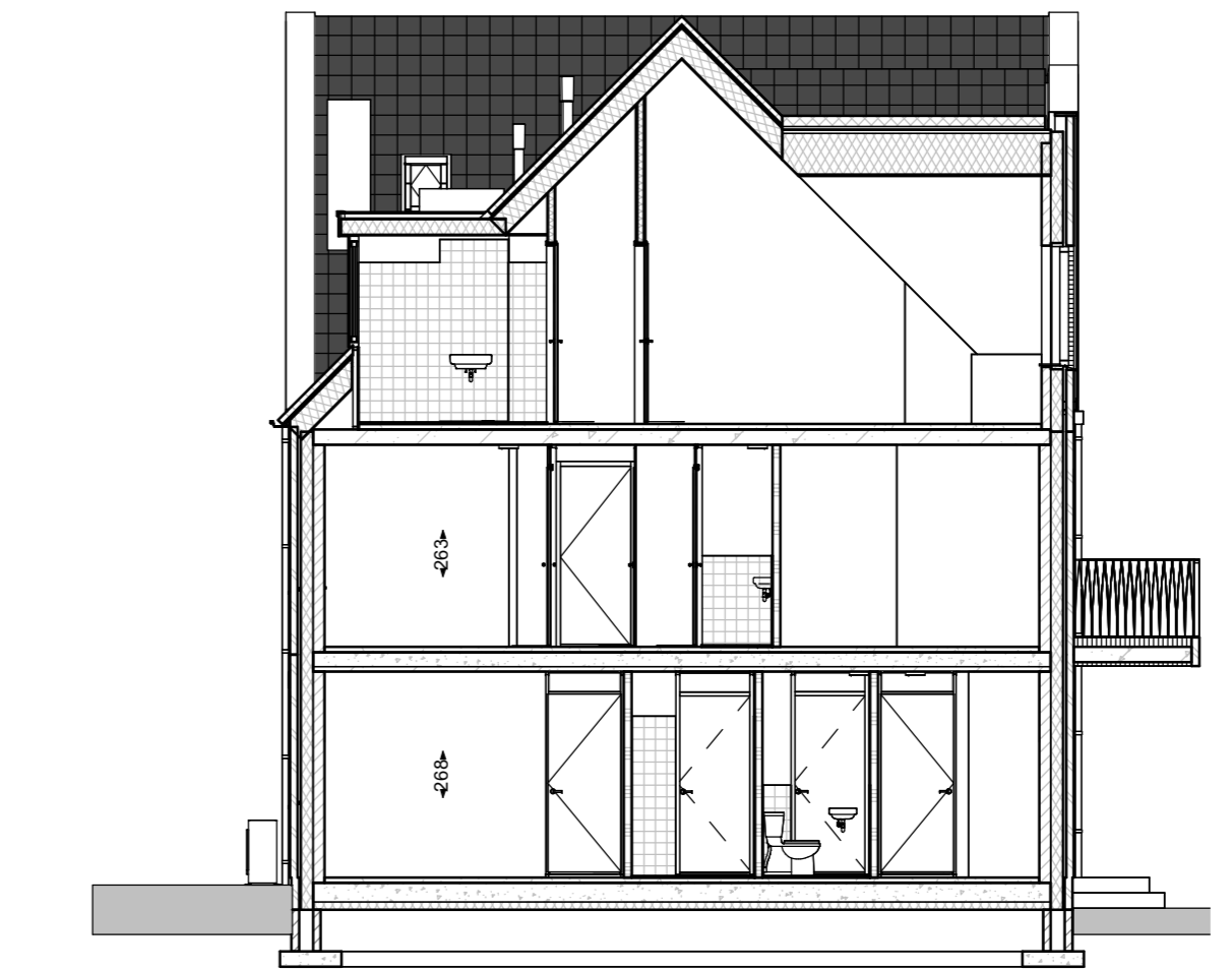
DOORSNEDE C schaal 1:100
