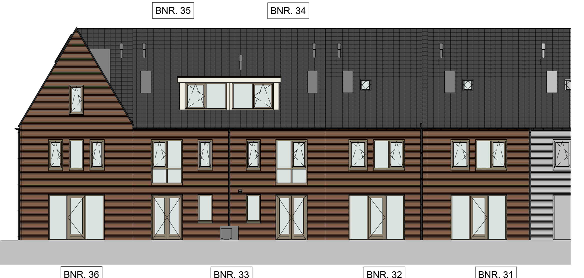
ACHTERGEVEL schaal 1:100
