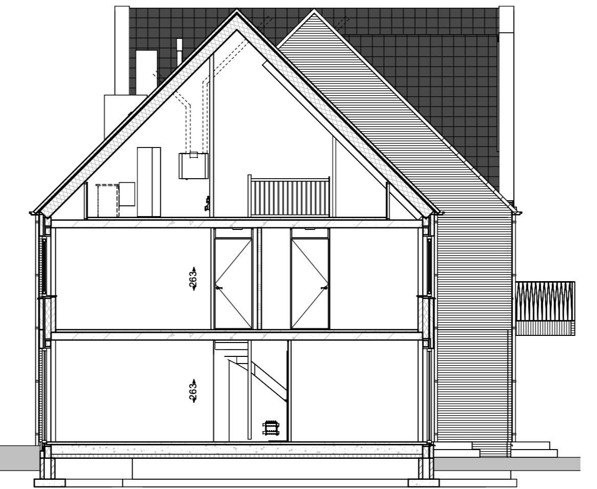
DOORSNEDE B schaal 1:100
