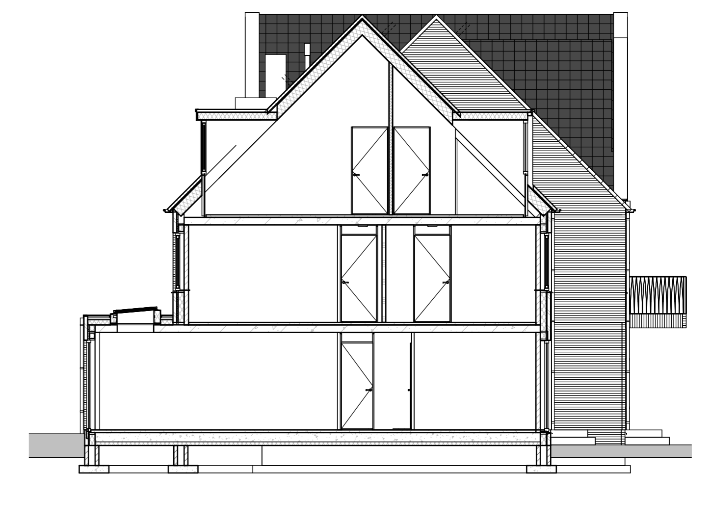
DOORSNEDE B schaal 1:100
