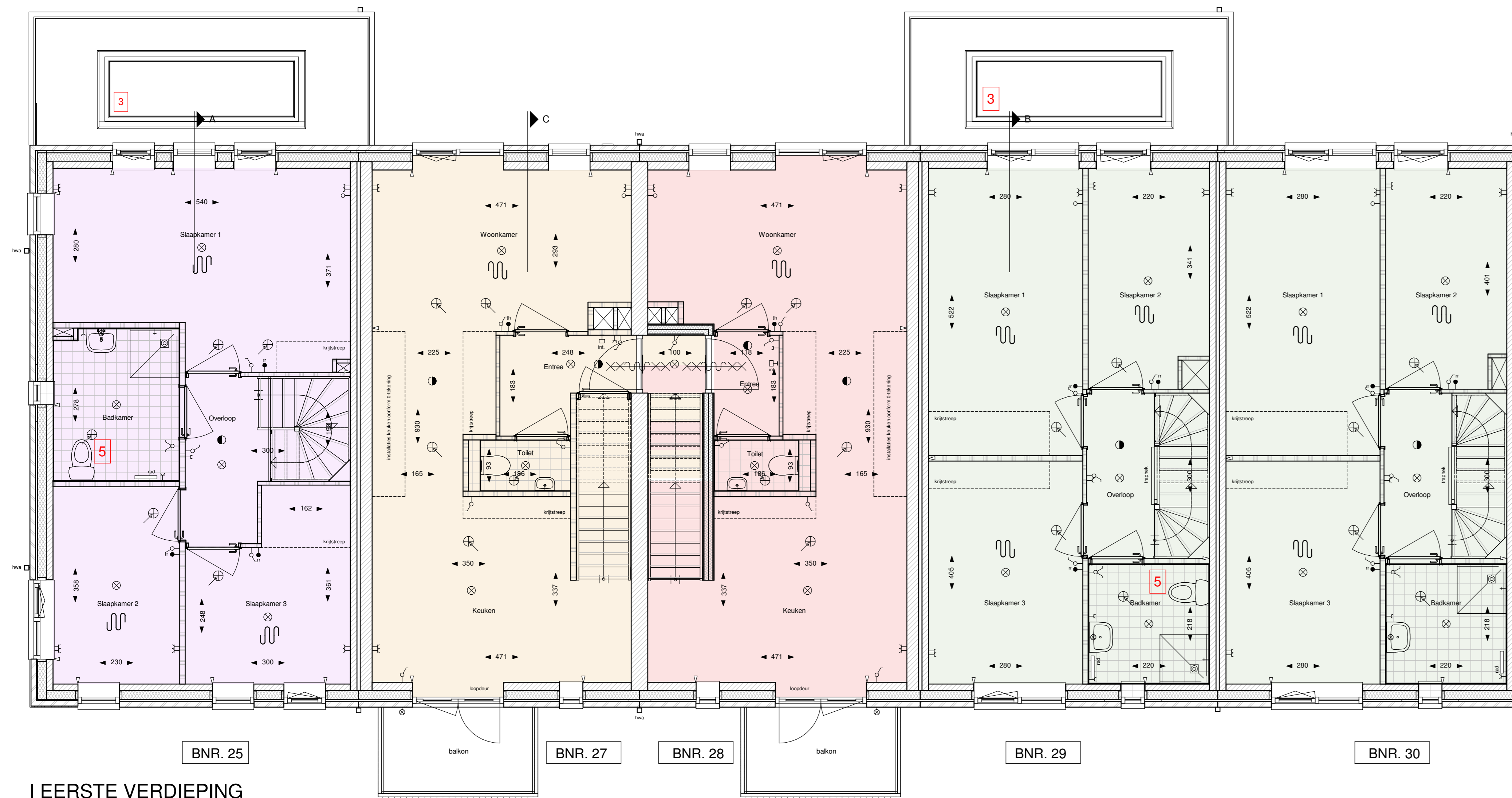
EERSTE VERDIEPING schaal 1:50
