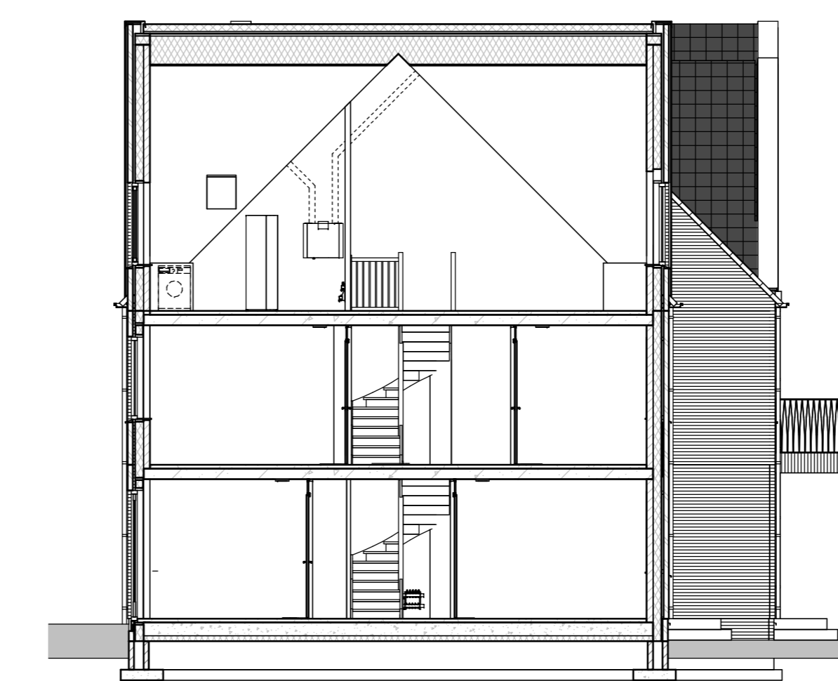
DOORSNEDE A schaal 1:100
