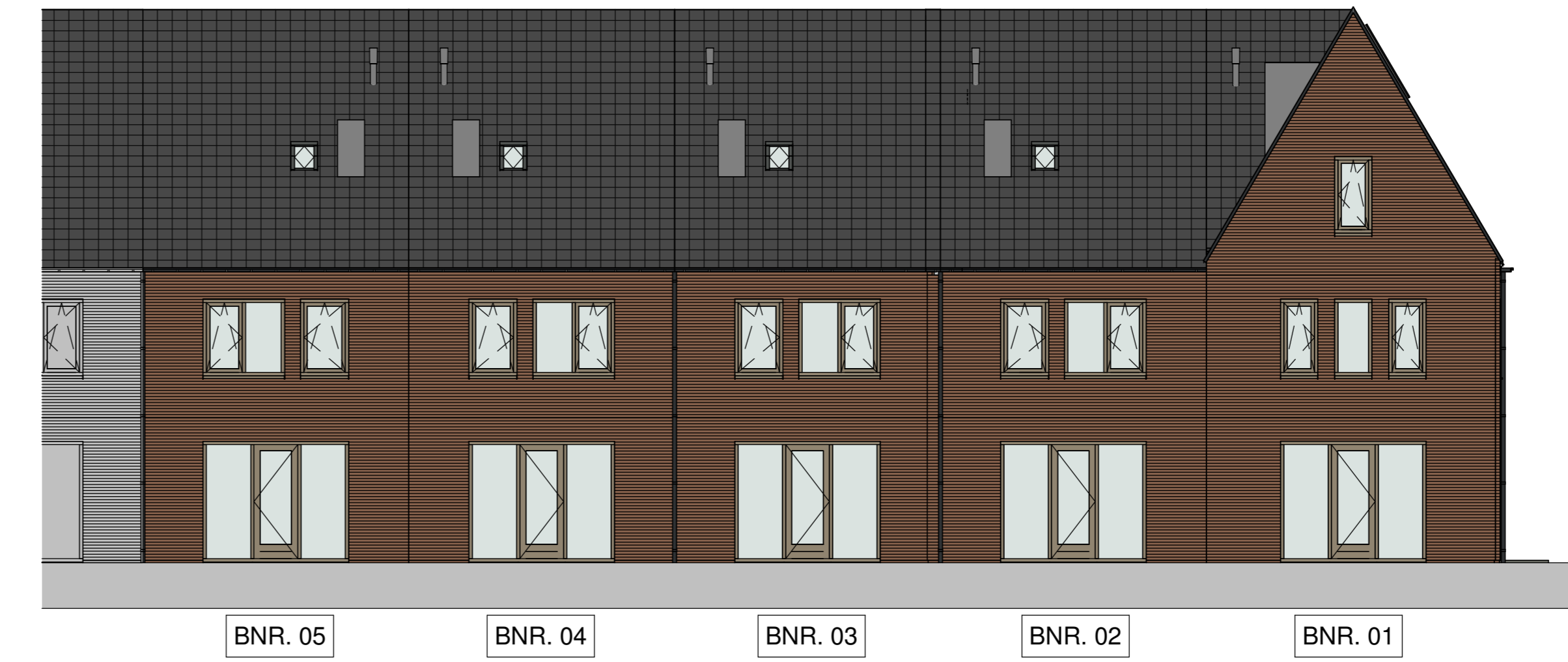
ACHTERGEVEL schaal 1:100
